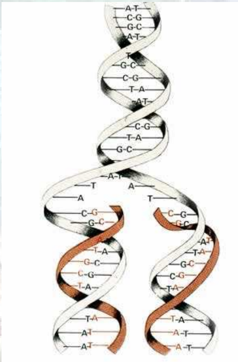
Fig. 24. 2 DNA
